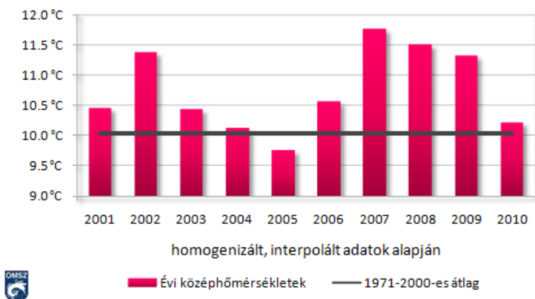
Országos évi középhőmérsékletek 2001-2010
