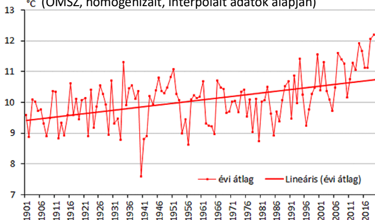
Az országos évi középhőmérsékletek 1901 és 2019 között °C (OMSZ, homogenizált, interpolált adatok alapján)
